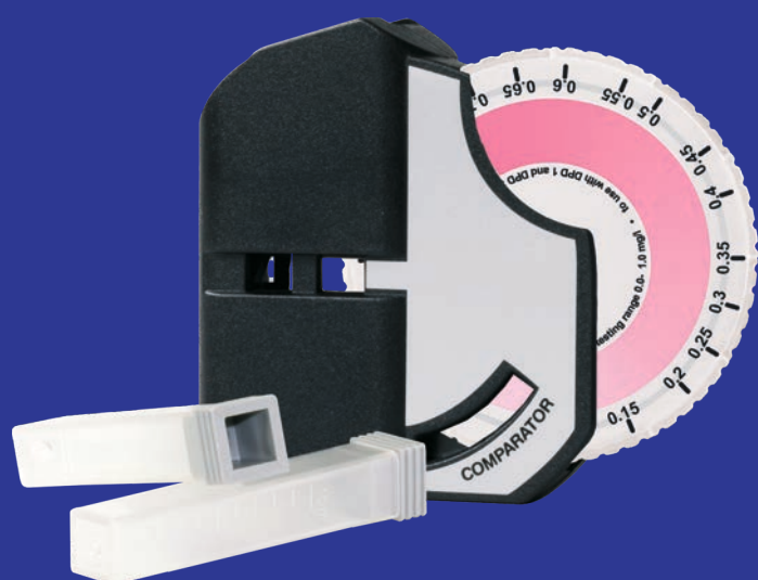
PCP001 с FD100 Компаратор Water-i.d. с диском Хлор 0.00 – 1.00 ppm
